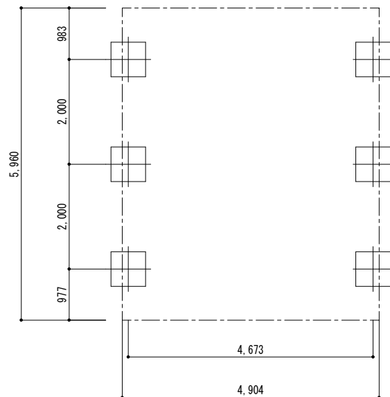
■ 基礎配置図
